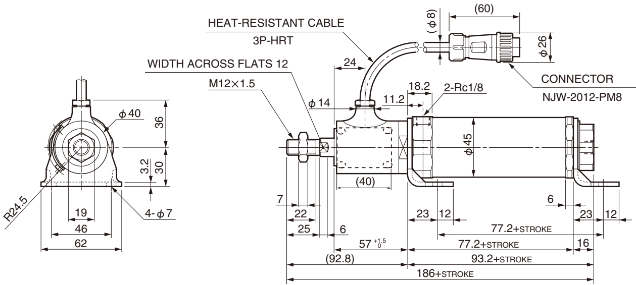
CSAH-40×□-LB
